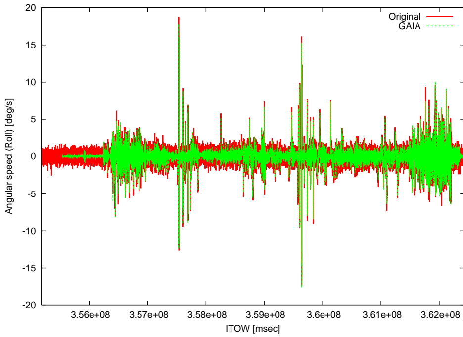
図4 ロール角速度
