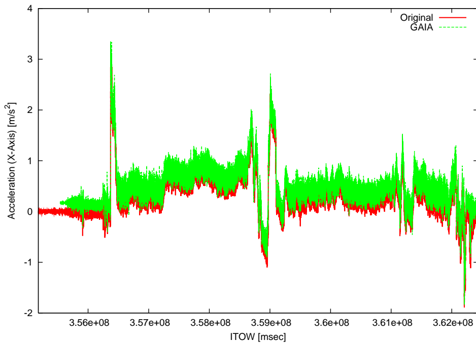
図1 X軸加速度
