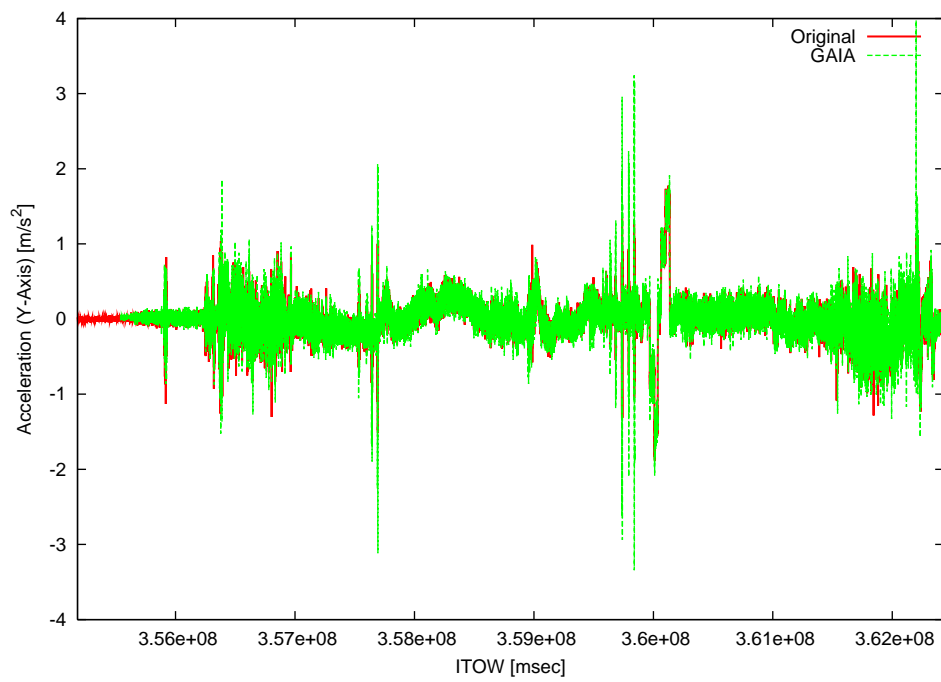
图 2 Y 轴 加速度
