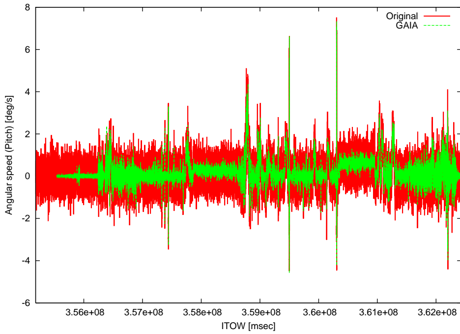
図5 ピッチ角速度
