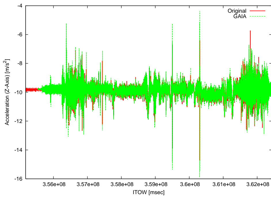
图 3 Z 轴 加速度
