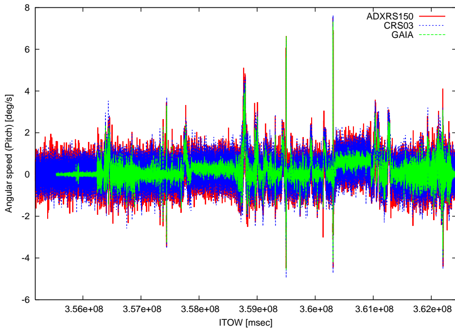
図2 ピッチ角速度
