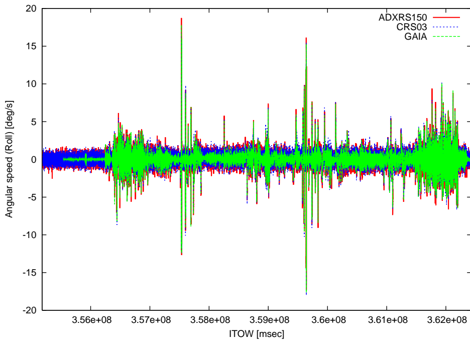
図1 ロール角速度
