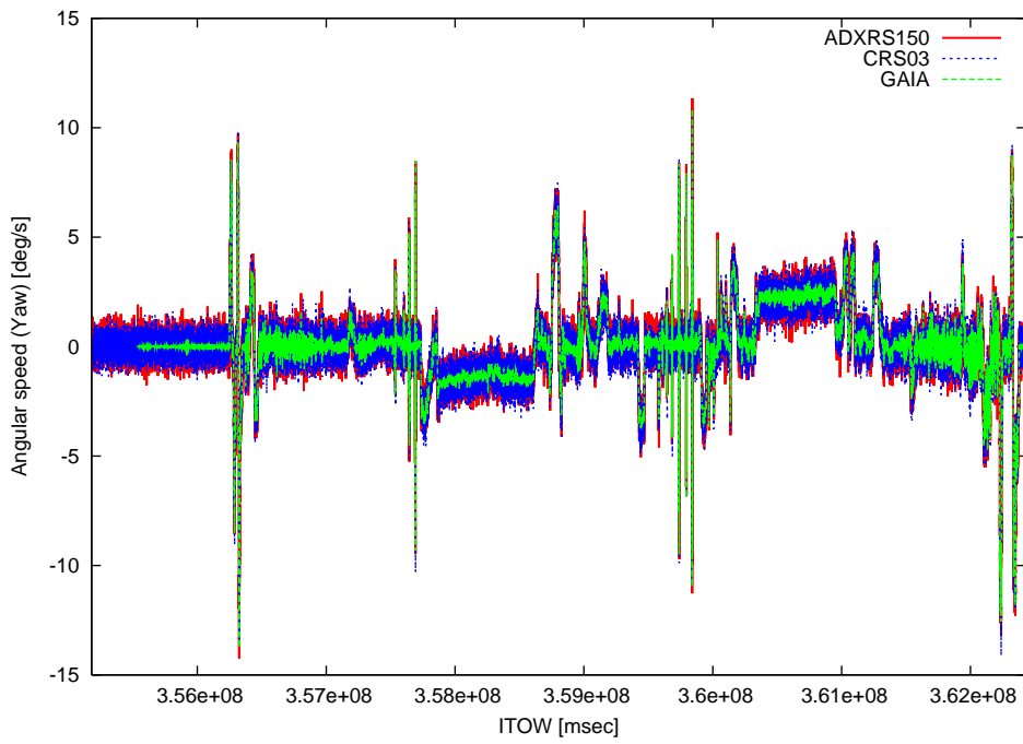
図3 ヨー角速度
