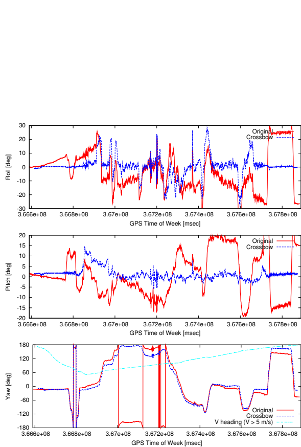
図3 姿勢履歴
