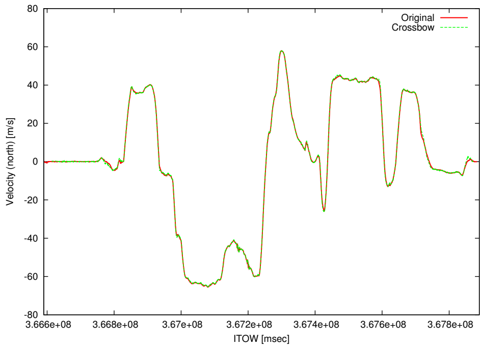
图 3 北方向速度
