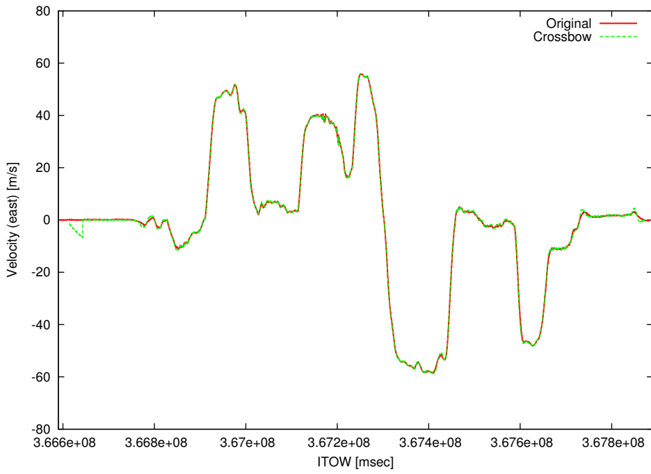
图 4 東方向速度
