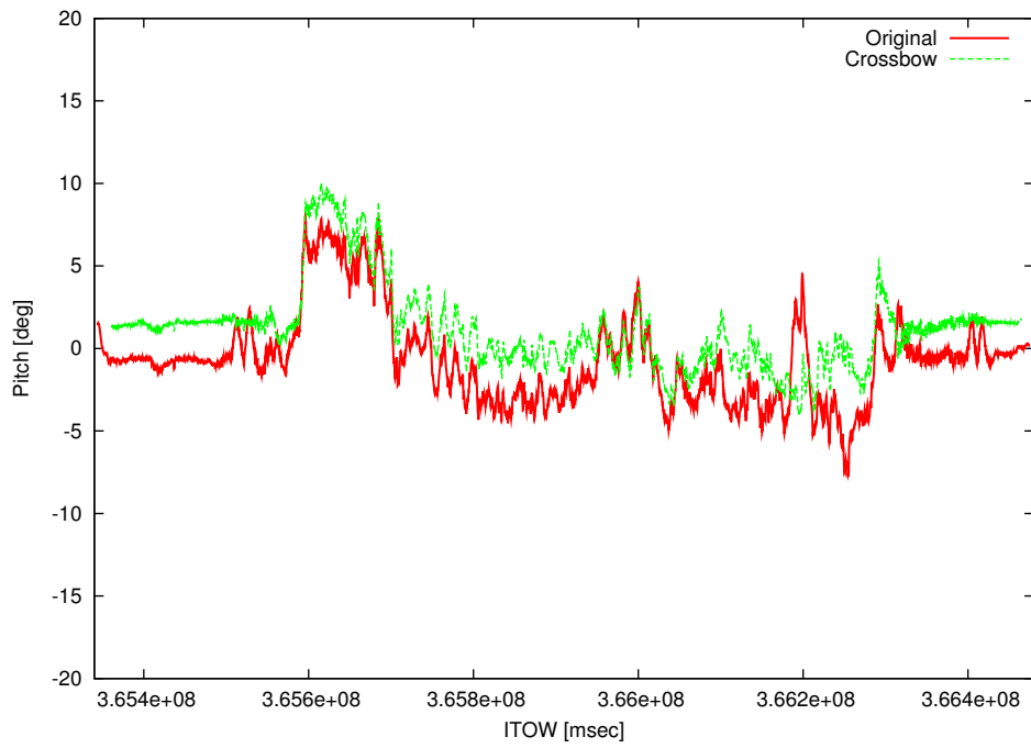
図7 ピッチ
