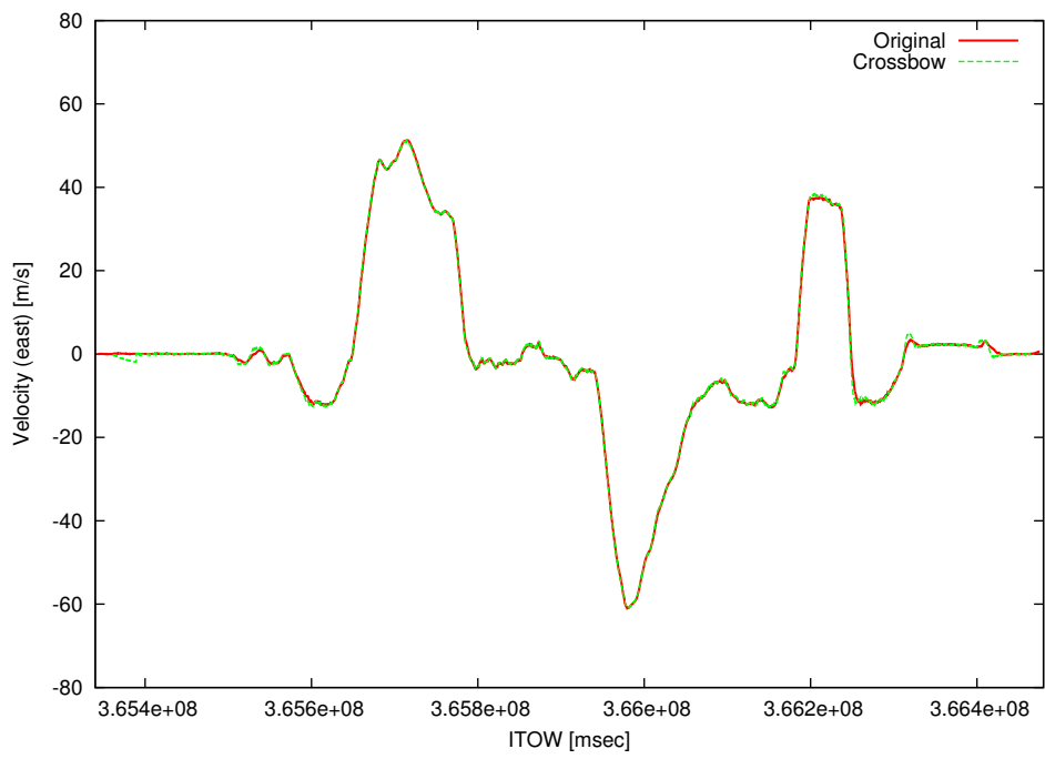
图 4 東方向速度
