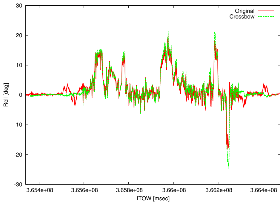
図6 ロール
