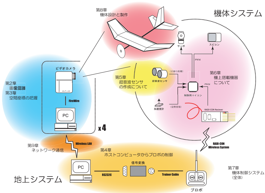
図2 開発すべき要素、ならびに搭載機器
