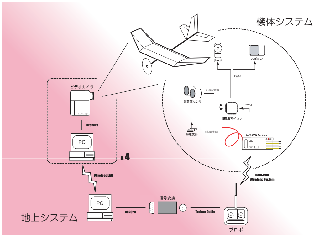
図1 システム全体
